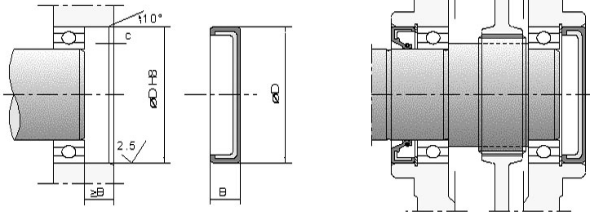
VK - уплотнение/крышка подшипникового узла
