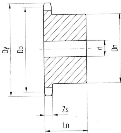
Ketjulle ISO-nr 05B-1 Jako 8 mm x 3 mm
